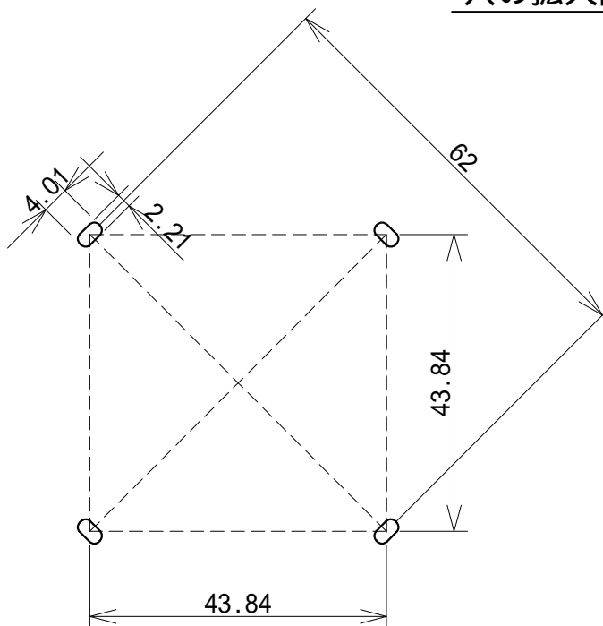
穴の拡大図
