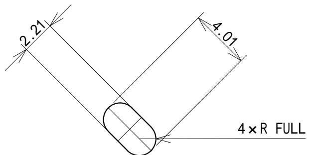
穴の拡大図
